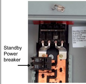
FIG. 2 Install Interlock
