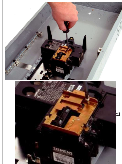
FIG. 2 Install Interlock
