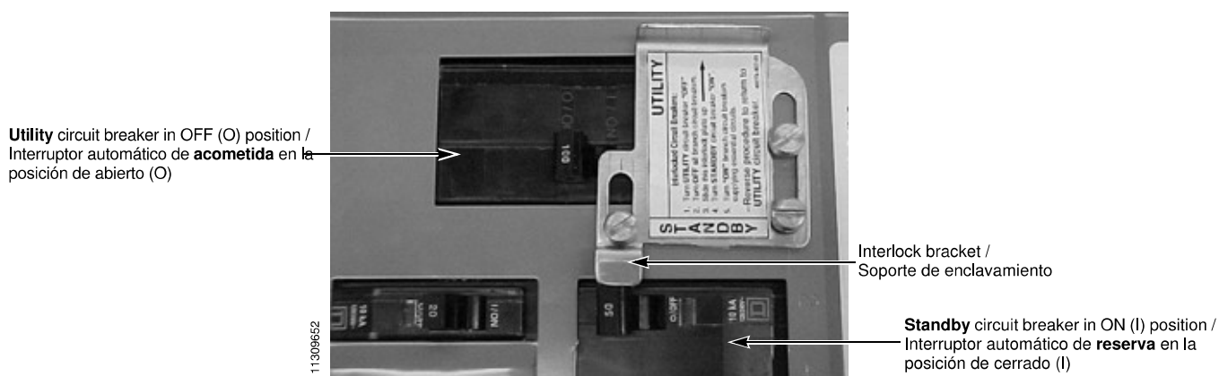
Figure / Figura 4: Utility Circuit Breaker in OFF (O) Position / Interruptor automático de acometida en la posición de abierto (O)
